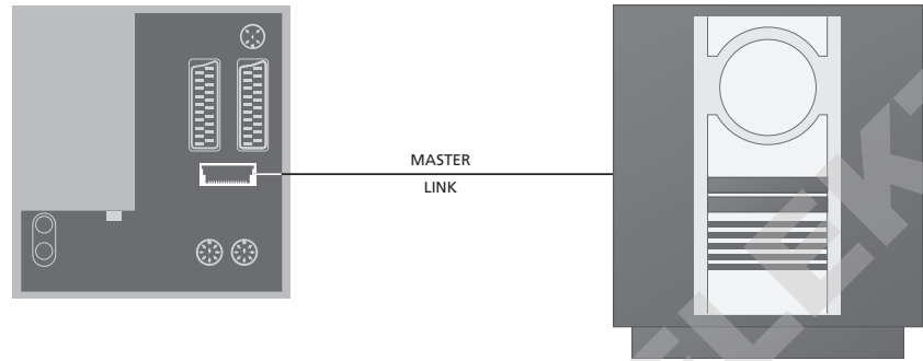
BeoVision 6
