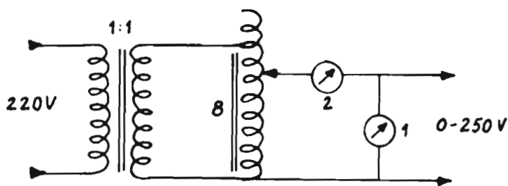
Fig. 2. Funktionsdiagram.
